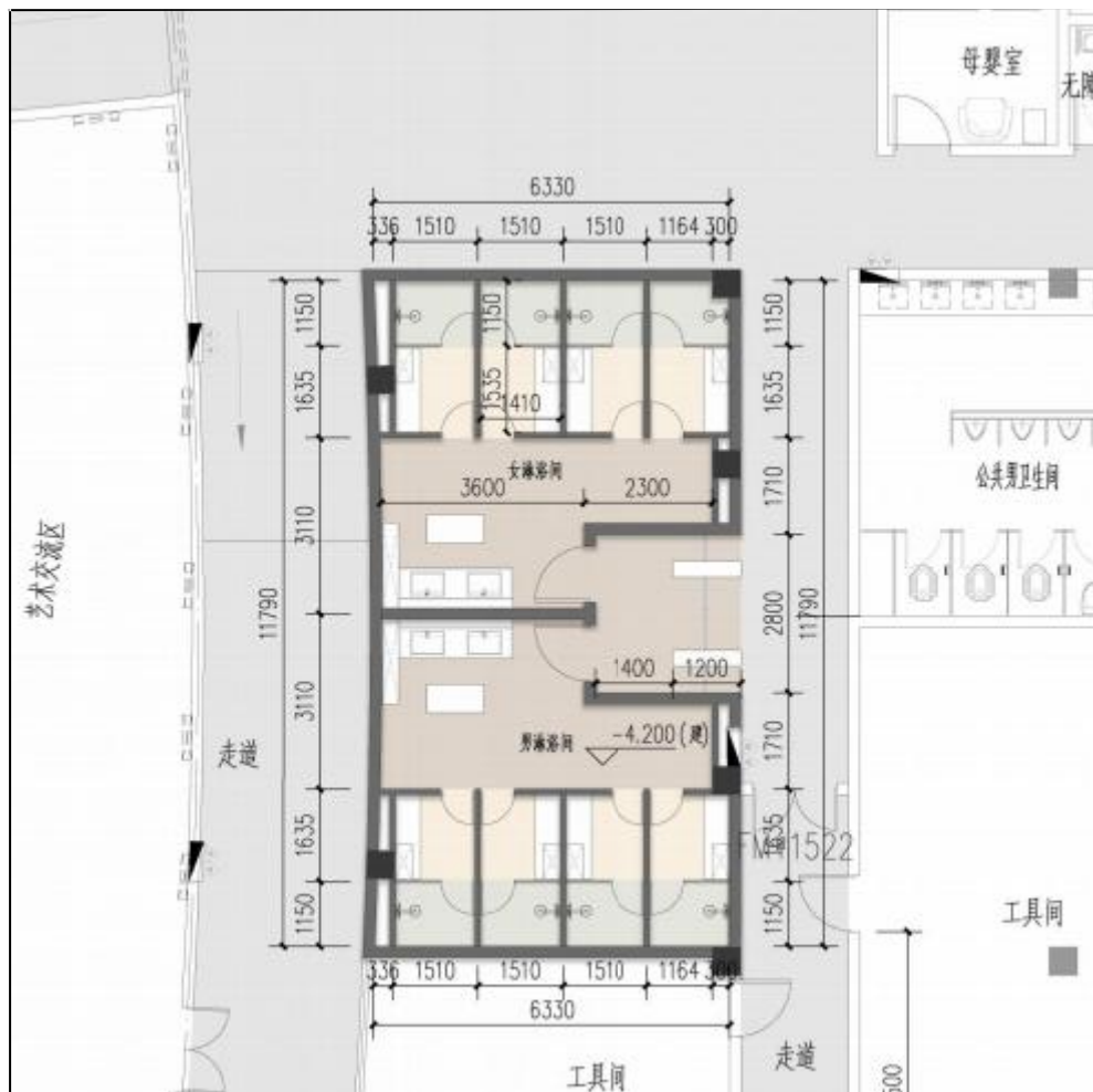
淋浴间平面图
